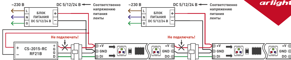
Рисунок 2. Подключение нескольких лент или лент с током потребления более 2 А.
