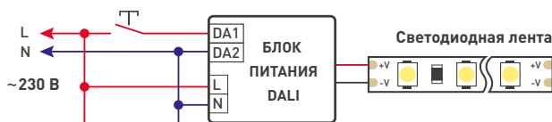
Рис. 1. Схема подключения при использовании внешней кнопки (Push Dim).
